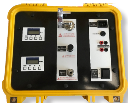
↳ Analyseur d'oxygène
