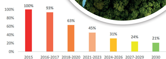
Évolution de la quantité de HFC disponible sur le marché, en Teq CO2
